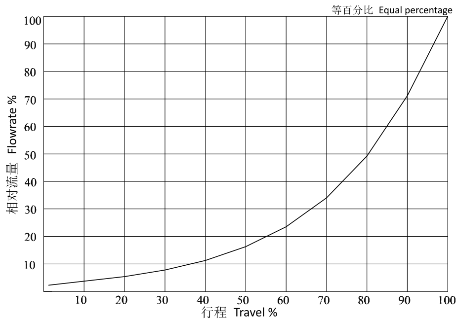
G150 系列控制阀流量特性曲线（等百分比、线性） G150 Series Control Valve Flow Characteristic Flow chart(Equal percentage/Linear)
